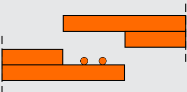
Proužky lepidla o průměru \varnothing 5 mm
