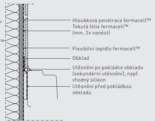
Napojení stěna – sprcha nebo vana, napojení na montovanou stěnu, jednovrstvé opláštění
