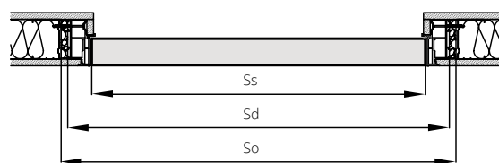
dveře ODZ (otevírání ven)
