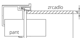
varianta 1 otevření ODZ směrem ven zrcadlo protilehlé k závěsům (A/Z)
