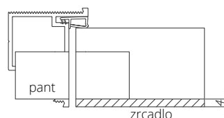
varianta 2 otevření směrem ven ODZ zrcadlo na straně závěsu (Z)
