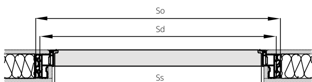
dveře ODW (otevírání dovnitř)
